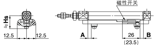
( )内数值表示D-A96型の場合。
