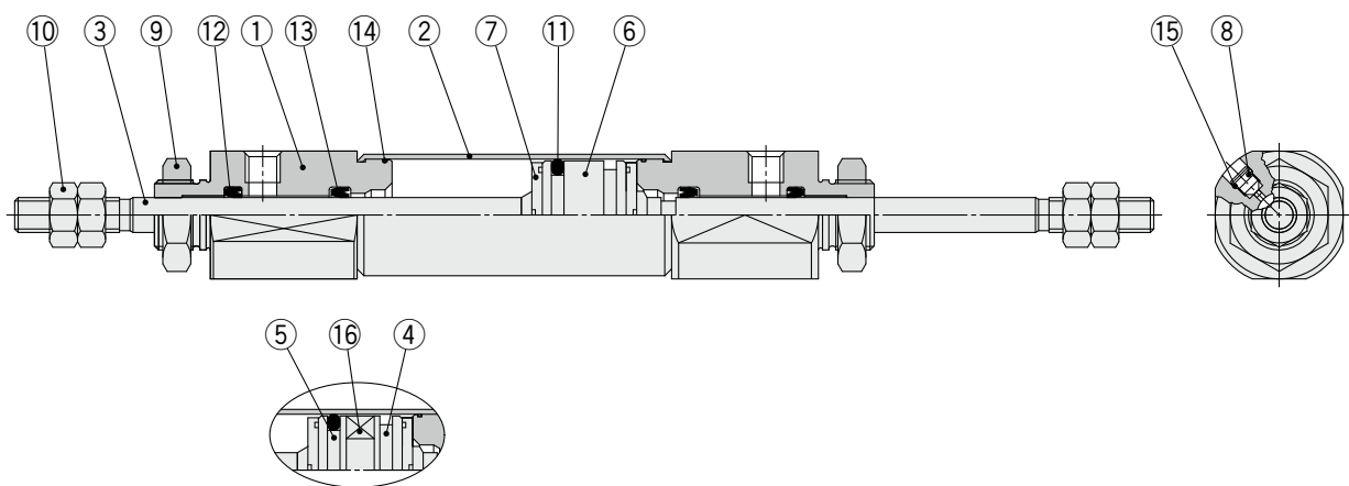
带磁性开关の場合
