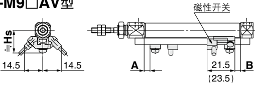
( )内数值表示D-M9□AV型の場合。
