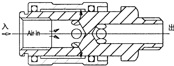
阀关闭
