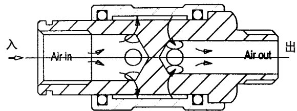
阀导通
