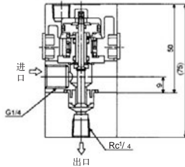
2通喷涂用阀
