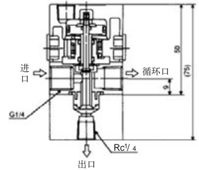
3通喷涂用阀
