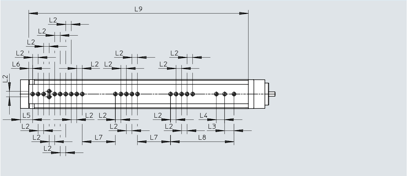
Dimensions – EGSL-55-250
