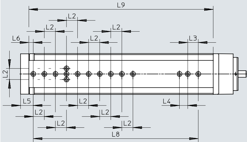
Dimensions – EGSL-75-200
