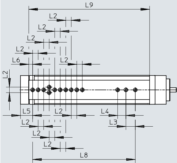
Dimensions – EGSL-55-100
