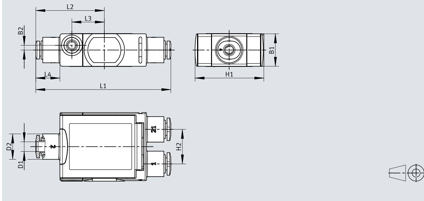
Dimensions – VBNF (inline)
