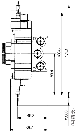
L型插座式
