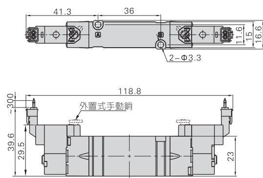
7MV120(先導閥M型)
