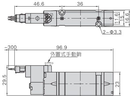
7MV110(先導閥JPC型)
