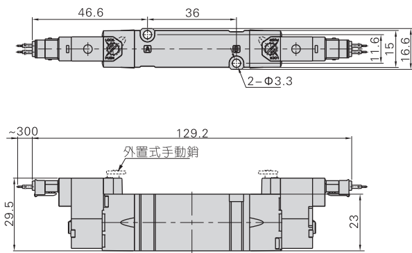
7MV120(先導閥JPC型)
