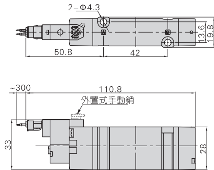
7MV210(先導閥JPC型)
