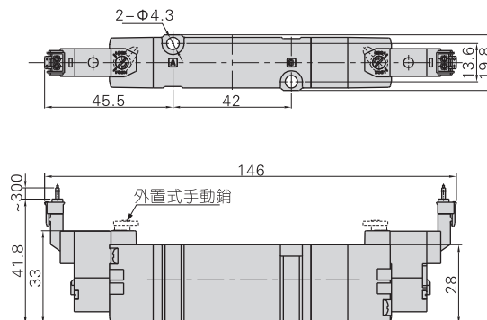
7MV230(先導閥M型)
