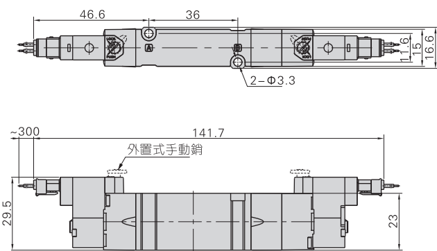
7MV130(先導閥JPC型)
