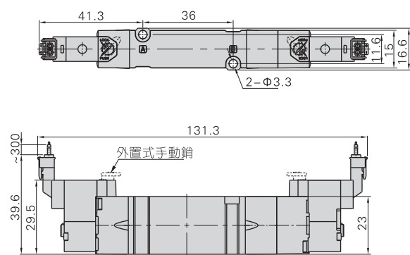
7MV130(先導閥M型)
