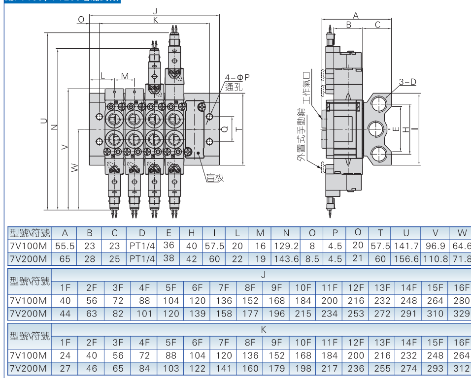
配7V100、7V200電磁閥類
