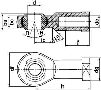
I型单肘节接头
