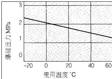
爆破压力特性图
