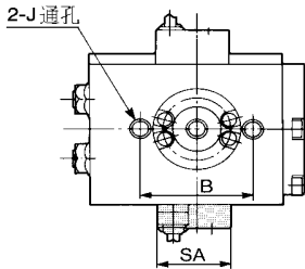
内置磁环系列 D-A7•A8•F7•F8型
