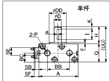
内置磁环型 Ø20•Ø30•Ø40
