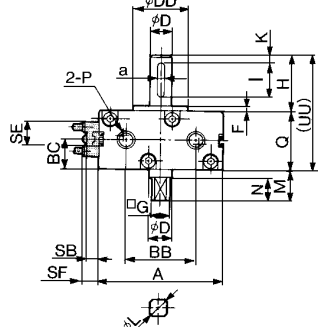
内置磁环连开关
