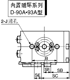
外形尺寸图（毫米）
