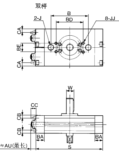
基本型 Ø20•Ø30•Ø40
