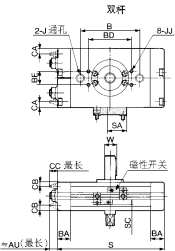
内置磁环型 Ø20•Ø30•Ø40
