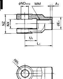
Y型双肘节接头
