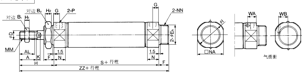
外形尺寸图（毫米）
