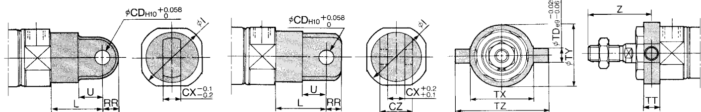
单U型钩
