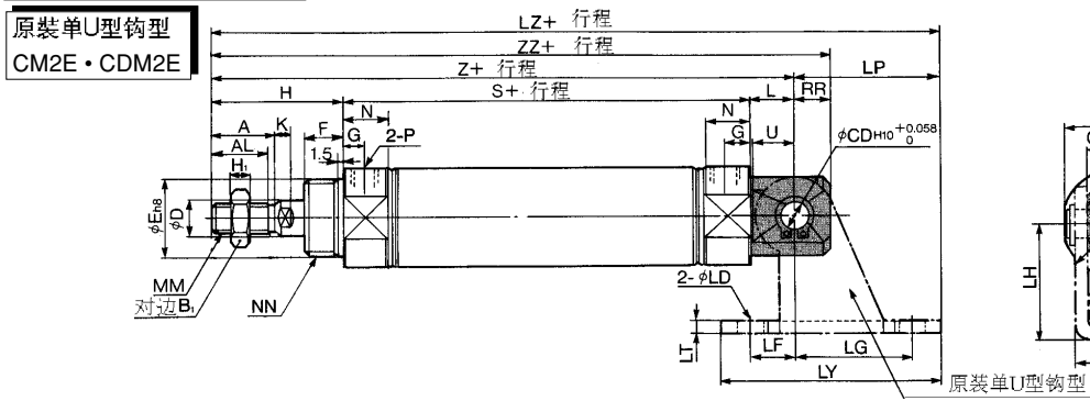
外形尺寸图（毫米）
