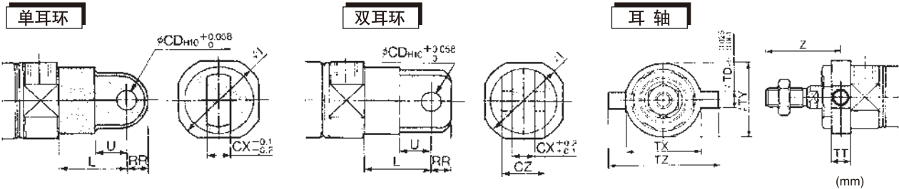
外形尺寸图（毫米）
