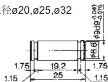
肘节接头用销子
