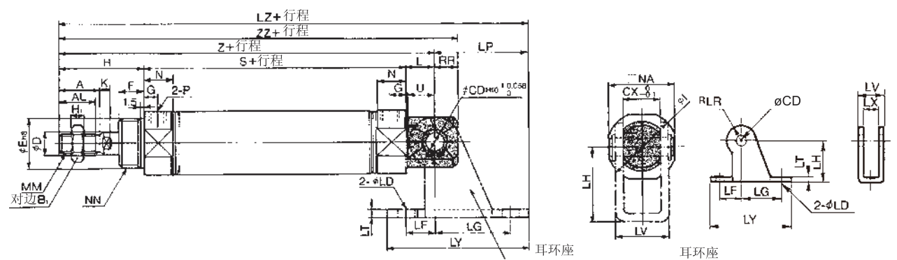
耳环一体型 CM2E-CDM2E
