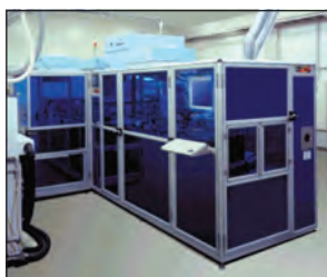
DVD 生产设备 (层合机) "DVD 碟 温度控制"
