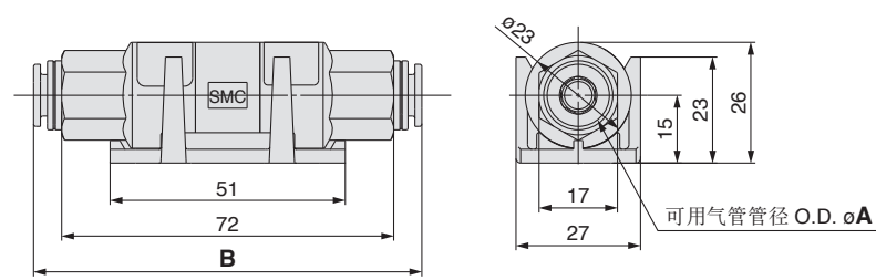
托架安装尺寸
