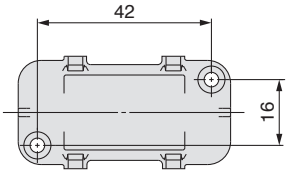
托架安装尺寸
