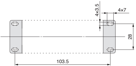
托架安装尺寸
