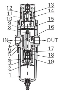
差壓排水式
