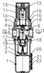
差壓排水式
