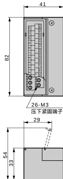
● 集中端子台 (压下紧固) T11
