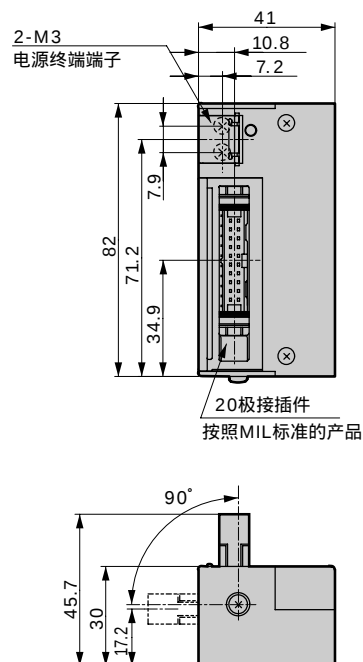
● 20针脚扁平电缆接插件 (带电源端子) T50
