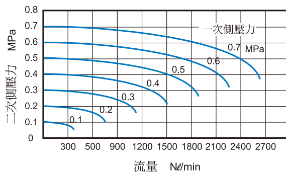
流量特性圖：
