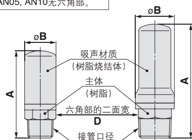
尺寸表 (mm)
