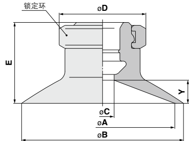
尺寸表
