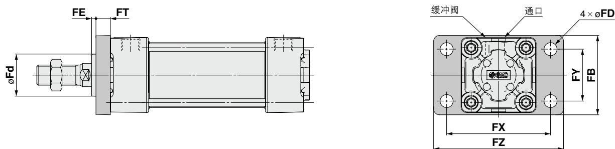
杆侧法兰型 (mm)
