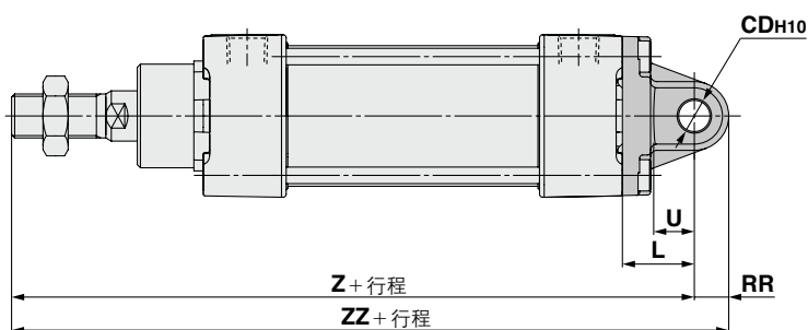
单耳环型 (mm)
