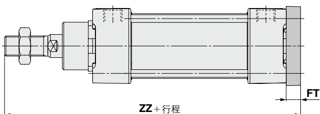
无杆侧法兰型 (mm)
