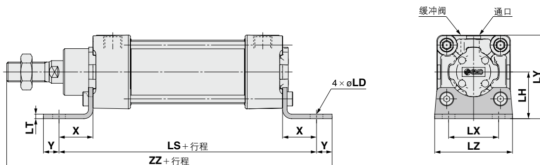
轴向脚座型 (mm)
