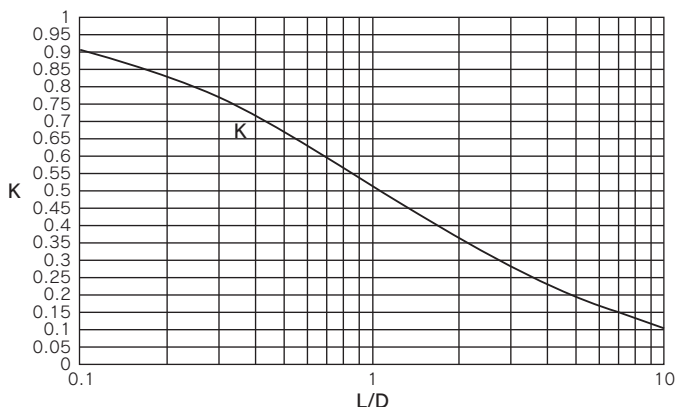
図1 クラウジング係数
