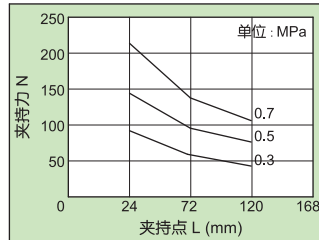
MHK40
