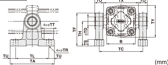
中间耳轴座
