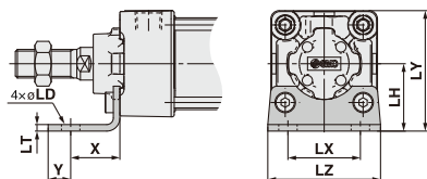
脚座
