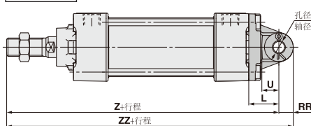
双耳环
