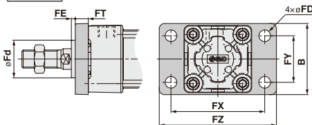
法兰
