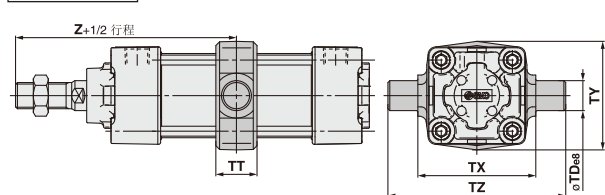
中间耳轴
