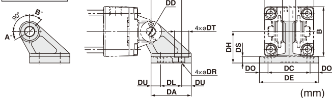
双耳环座
