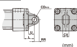
单耳环
