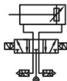
带阀型三位中排式
