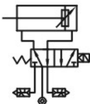
带阀型通电时推式
