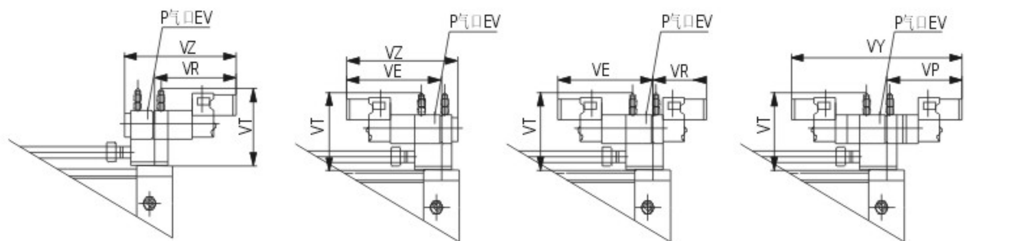
通电时推式
