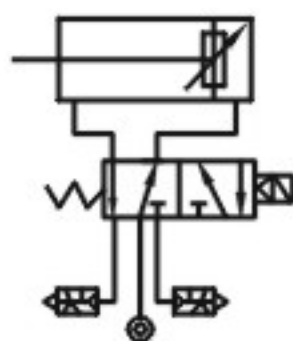
带阀型通电时拉式
