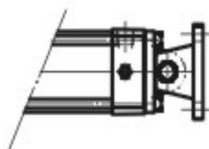
5、单悬耳座式 (HCA-CB)
