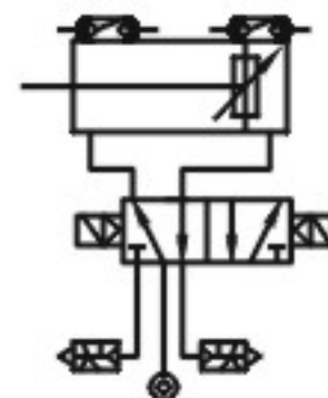
带阀带开关型
