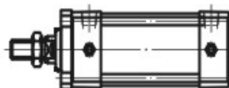
4、FA (前法兰式)
