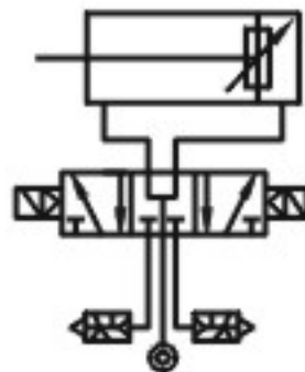
带阀型三位中压式
