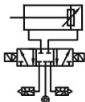
带阀型三位中封式样
