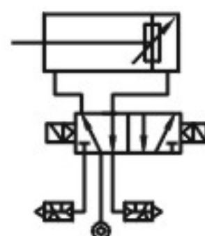
带阀型自己保持式
