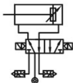
带阀型
