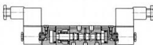
三位五通双电结构原理图（中封）
