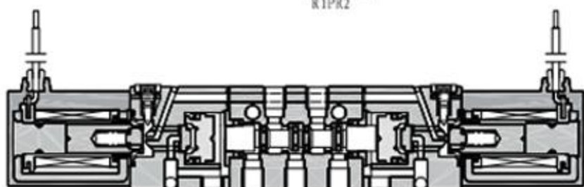
两位五通双电结构原理图
