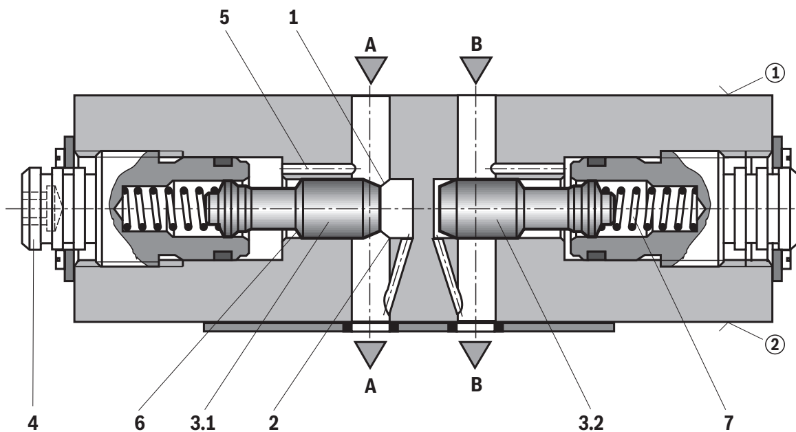
Zulaufdrosselung
