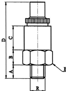
尺寸圖
