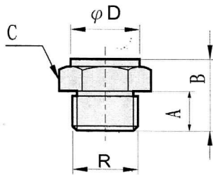
尺寸圖
