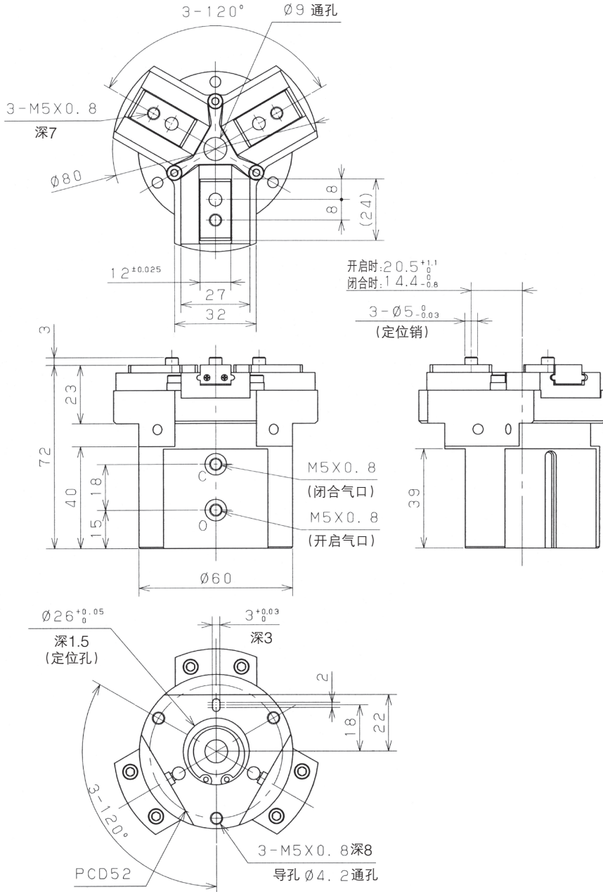
外形尺寸图 HP15-25C
